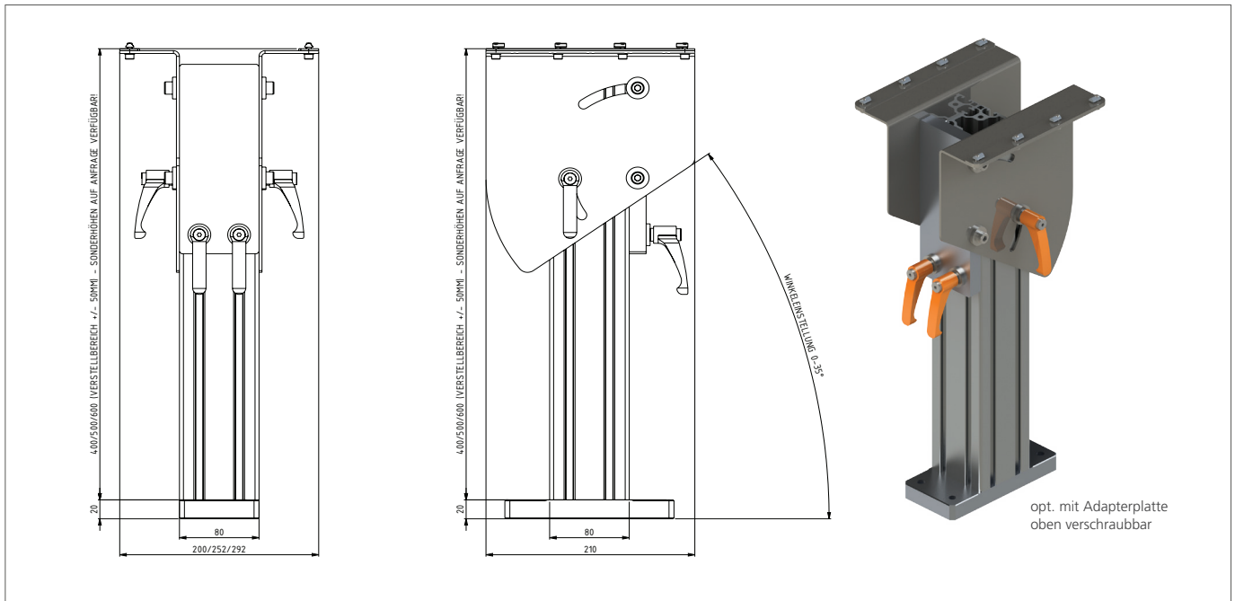
Montagestativ (Winkel und Höhe einstellbar)
