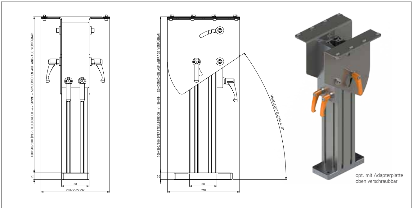
Montagestativ (Winkel und Höhe einstellbar)
